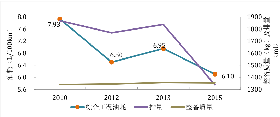
图 26 福特福克斯油耗、整备质量及排量变化
