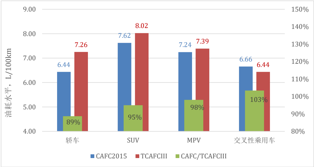
图 19 各类汽车产品平均油耗水平及达标情况
