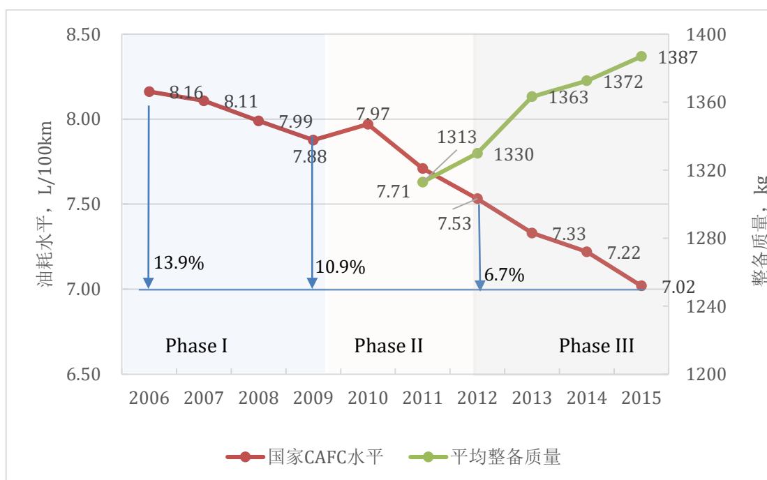
图 14 2006-2015 年国家乘用车油耗水平与整备质量发展趋势
