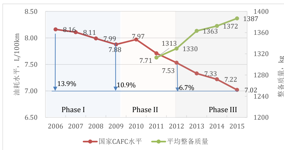
2006-2015 年国家传统乘用车油耗水平与整备质量发展趋势
