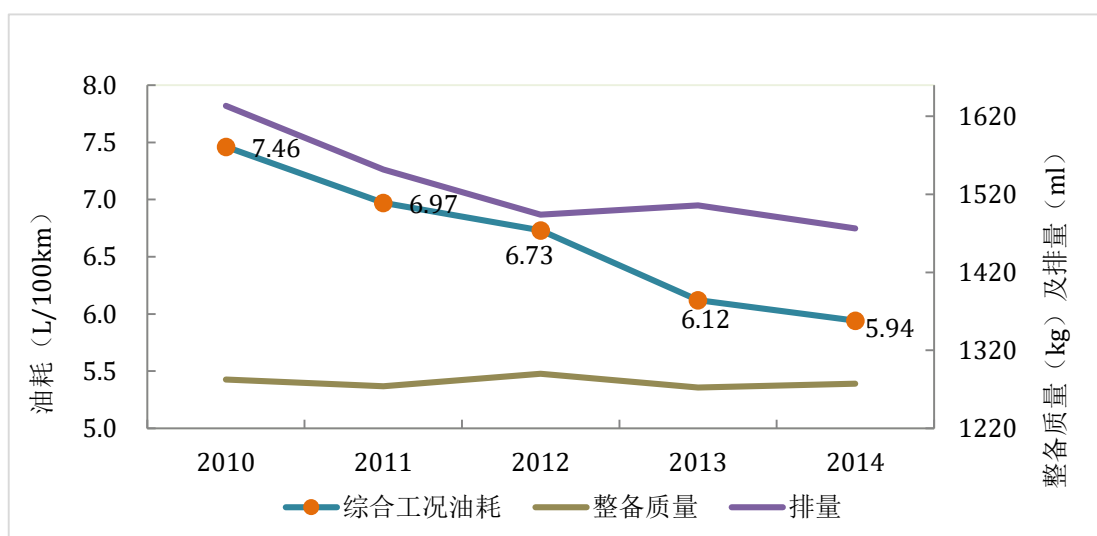
图 24 大众朗逸油耗、整备质量及排量变化
