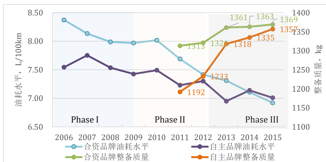
2006-2015 年合资与自主品牌乘用车油耗水平与整备质量变化趋势
