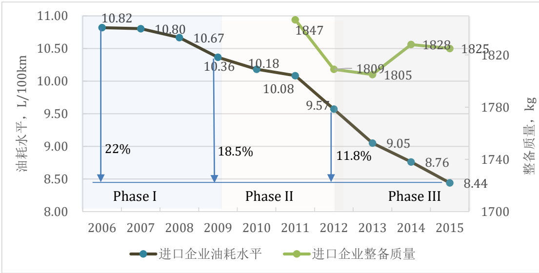
图 20 2006-2015 年进口车 CAFC 与整备质量变化趋势
